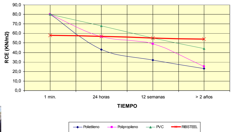
RIGIDEZ EN EL TIEMPO (NORMA DIN 16961)
